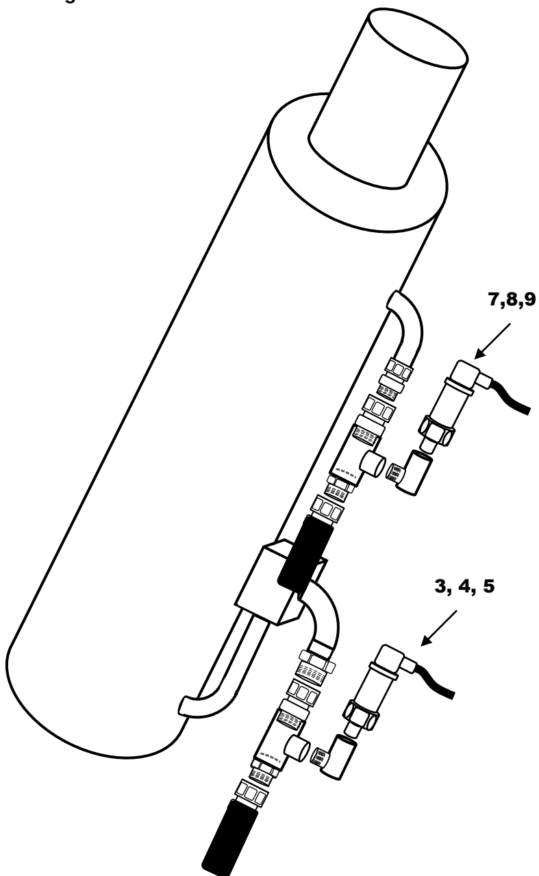
Fig. 2: implantation des capteurs de pression sur le vérin de levage
